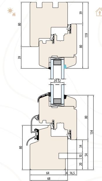
SISTEMA NATURO 68 Scanalatura per davanzale interno
