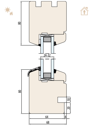
SISTEMA NATURO 68-FIX Scanalatura per davanzale interno
