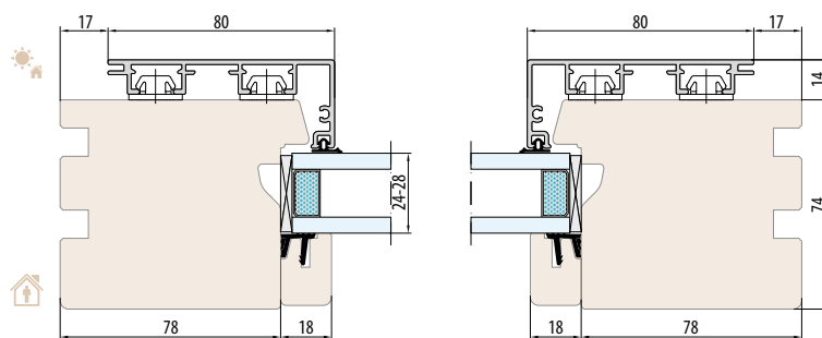
SISTEMA ESPERIA LIFE 74 ALU-Fix SEZIONE ORIZZONTALE B-B
