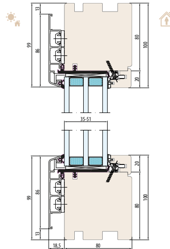
SISTEMA NATURO 80 ALU-FIX GEMINI CLASSIC Senza scanalatura per il davanzale
