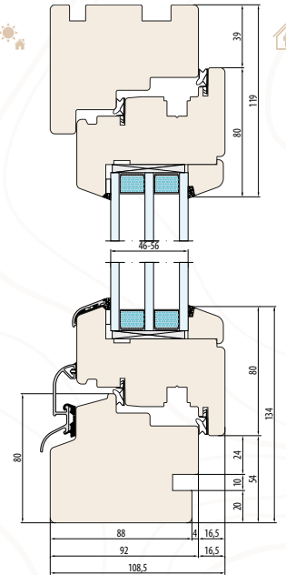
SISTEMA NATURO 92 Scanalatura per davanzale interno
