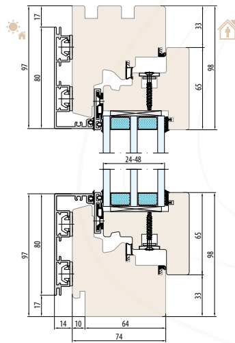
SISTEMA ESPERIA LIFE 74 ALU Scanalatura per davanzale esterno
