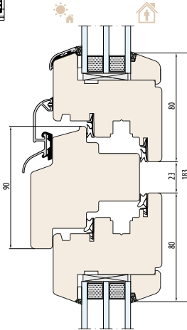
SISTEMA NATURO 80 Traverso 90 mm
