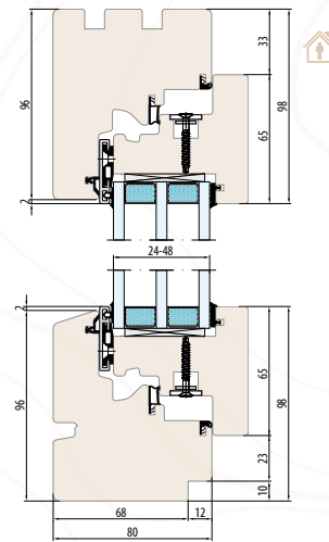
SISTEMA ESPERIA LIFE 80 Scanalatura per davanzale interno
