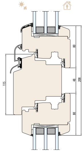
SISTEMA NATURO 92 šlemiję 115 mm
