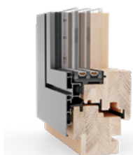
Gemini Quadrat FB Profilo standard (con scanalatura)
