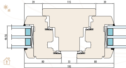
SISTEMA NATURO 92 Montante fisso 115 mm (Sezione orizzontale)
