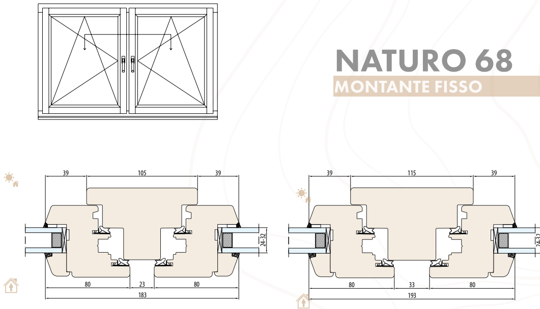
SISTEMA NATURO 68 Montante fisso 105 mm (Sezione orizzontale)
