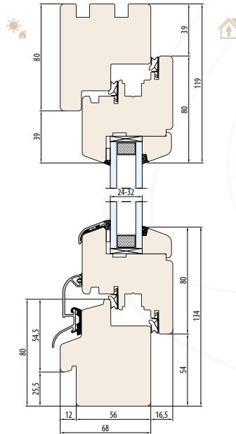
SISTEMA NATURO 68 Scanalatura per davanzale esterno
