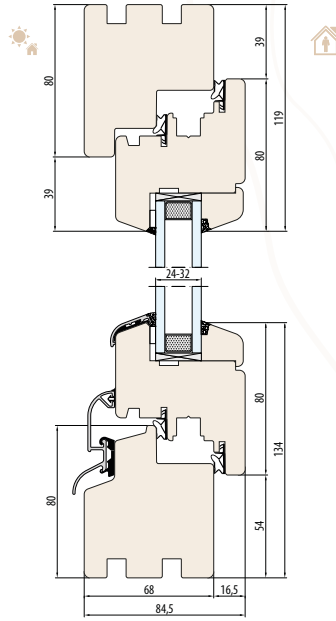
SISTEMA NATURO 68 Senza scanalatura per il davanzale
