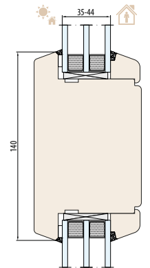
SISTEMA NATURO 80 Montante strutturale 140 mm
