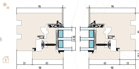
SISTEMA ESPERIA LIFE 80 SEZIONE ORIZZONTALE B-B
