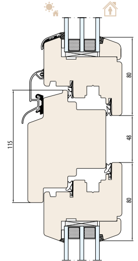
SISTEMA NATURO 80 Traverso 115 mm
