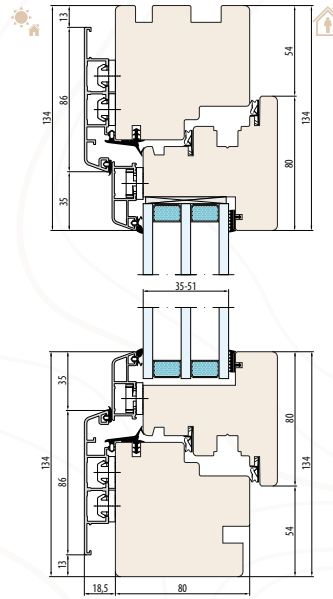
SISTEMA NATURO 80 ALU GEMINI CLASSIC Scanalatura per davanzale interno
