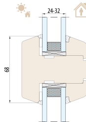
SISTEMA NATURO 68 Montante strutturale 68 mm
