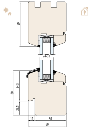
SISTEMA NATURO 68-FIX Scanalatura per davanzale esterno
