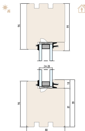
SISTEMA ESPERIA LIFE 80-Fix Senza scanalatura per il davanzale
