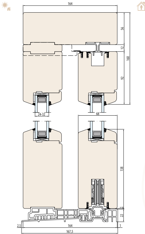
SISTEMA NATURO 68 HST (Dimensioni generali) - soglia 22 mm - schema "A"
