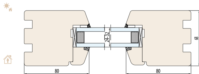
SISTEMA NATURO 68-FIX SEZIONE ORIZZONTALE B-B
