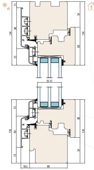
SISTEMA NATURO 80 ALU GEMINI CLASSIC Scanalatura per davanzale esterno
