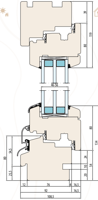
SISTEMA NATURO 92 Scanalatura per davanzale interno ed esterno
